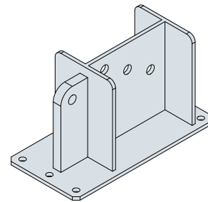
Herraje de arriostramiento
